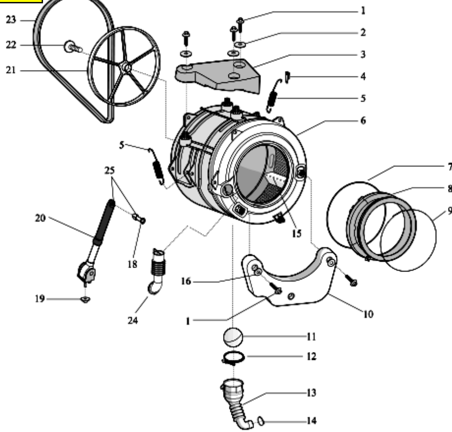
VUE B
